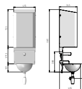
LMO-CE commande optique
